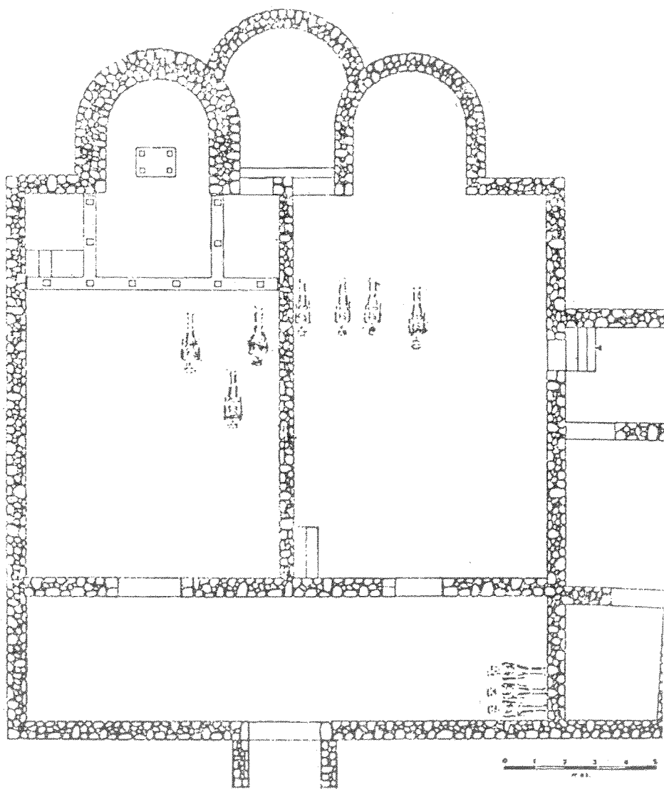
Slika 1. Tloris crkve u Bilimišću kod Zenice (prema Đ. Basleru)
