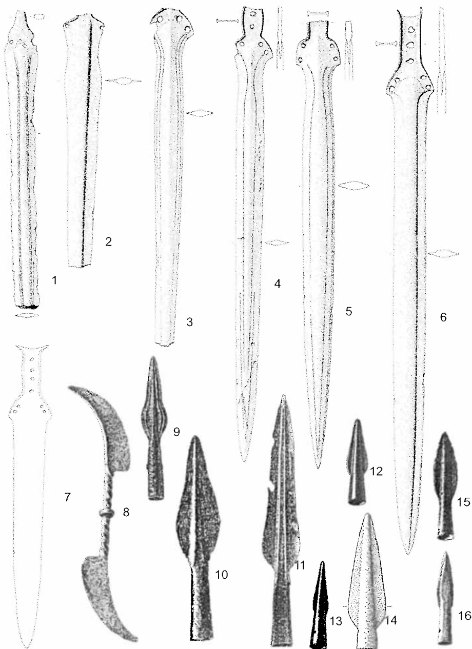
Taf. 3. 1 Donji Kamengrad ; 2 Pridražić ; 3 Hrbljina ; 4 Zvornik, Radeljska Ada ; 5 Buzija ; 6 Antonići ; 7 Fundort unbekannt, Fluß Sava ; 8 Lašva ; 9 Crna Rijeka ; 10 Očigrije ; 11 Mostarsko Blato ; 12 Tasovčići ; 13 Tešanj ; 14.15 Livno ; 16 Ljubuški (1–7 nach Harding; 8.16 nach Radimský; 9.11 nach Čurčić, 10 nach Nikolić; 12.13 nach Truhelka; 14 nach Marović; 15 nach Mandić); 1:4.
