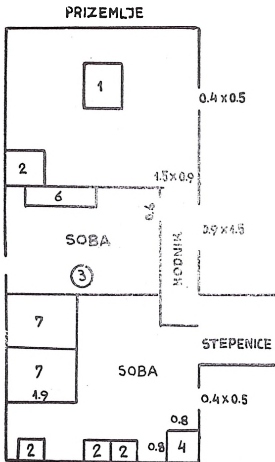
Sk. 43 a. Tlocrt kuće-čardaka — Selima Krhana iz Kričanja.
