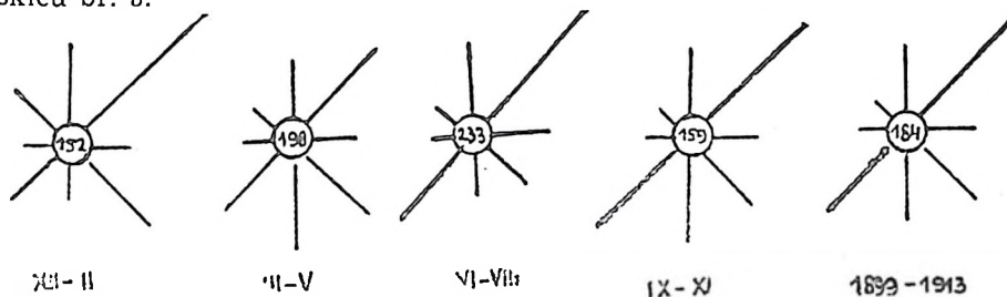
Sk. 5. Čestina vjetra po godišnjim dobima — petnaestogodišnji prosjek
