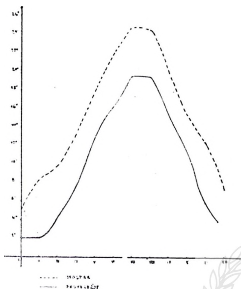
Sk. 1. Godišnje kretanje srednjih mjesečnih temperatura u Podveležju i u Mostaru u periodu od 1899 do 1913 god. zaključno.
