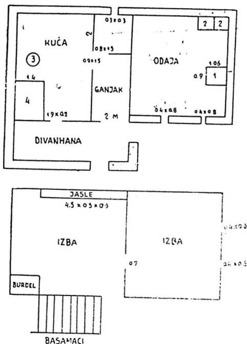
Sk. 38. Tlocrt kuće Osmara Gaste iz Opina.
