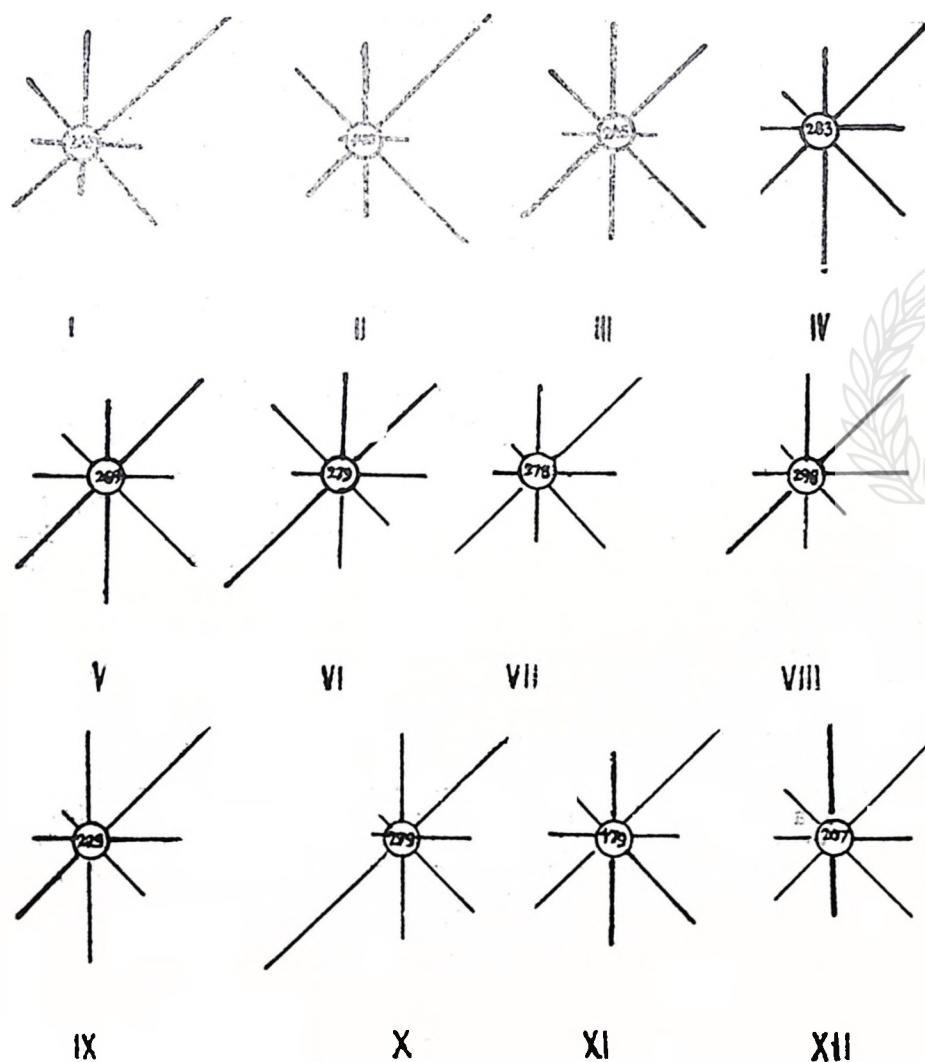
Sk. 4. Ruže vjetrova Podveležja po mjesecima. Period 1899 do 1913 zaključno
