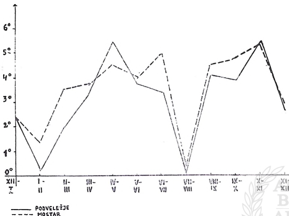
Sk. 2. Apsolutna promjenljivost srednjih mjesečnih temperatura u Podveležju i u Mostaru
