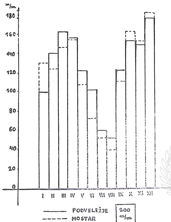
Sk. 8. Uporedni grafikon količina padavina po mjesecima u Podveležju
