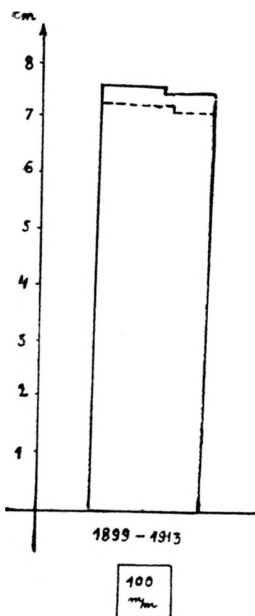
Sk. 6. Uporedni grafikon prosječne godišnje količine padavina u Podveležju i u Mostaru u periodu od 1899 do 1913 god. zaključno.
