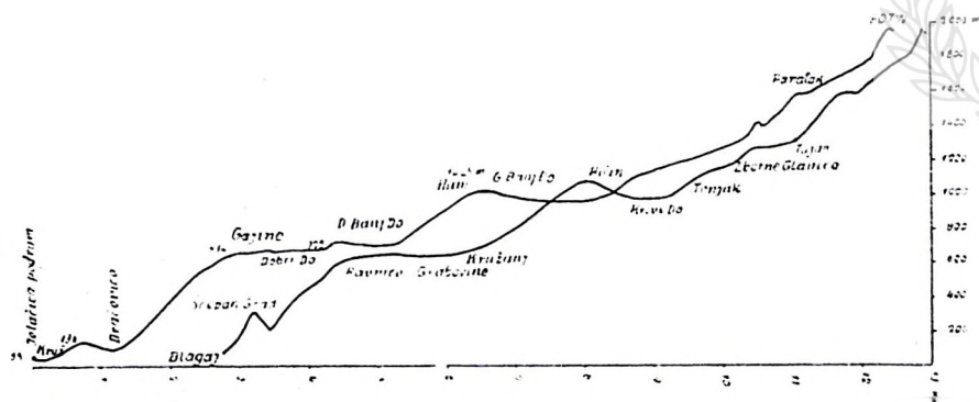
Presjek kroz Podveležje između Jelačića podruma i Botina te Blagaja i Botina
