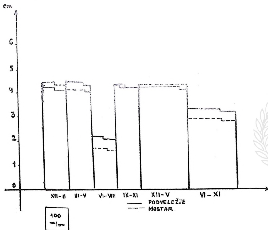
Sk. 7. Sezonsko kretanje srednjih količina padavina u Podveležju i u Mostaru u periodu od 1899 do 1913 god.
