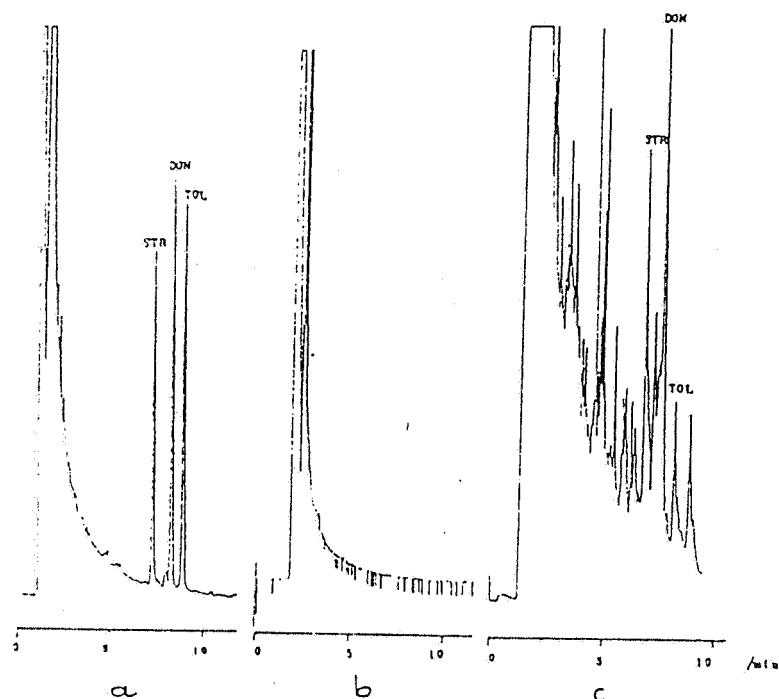
Slika 1. Kromatogrami a) standarda STR, DON i TOL b) zdravog kukuruza c) plesnivog kukuruza
