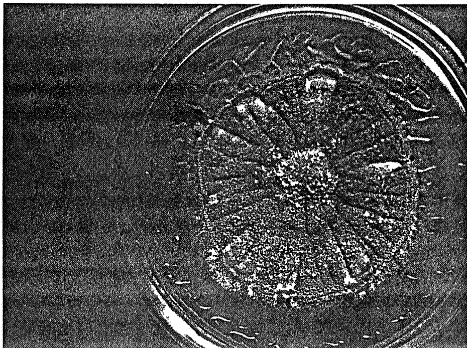
Sl. 2 – Karakterističan oblik kolonije A. versicolor : nepravilno, radijalna izbrazdana kolonija sa pahuljičastim centrom i baršunastim rubovima, nakon 20 dana na cropek podlozi
