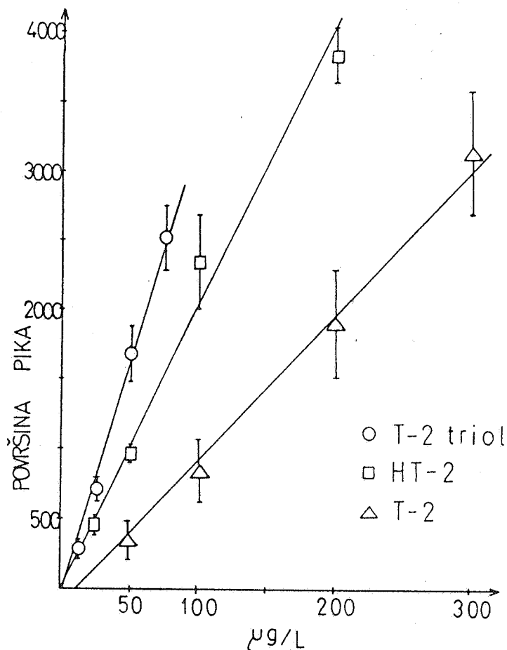
Sl. 3. Baždarni dijagrami za određivanje T-2 toksina, HT-2 toksina i T-2 triola u serumu. Rasponi označavaju standardnu devijaciju. Korelacioni koeficijenti: \circ r=0,9880 , \square r=0,9925 , \triangle r=0,9579
