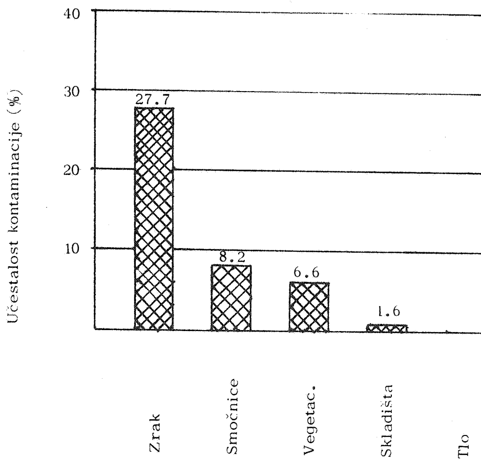
Graf.2. Učestalost A. versicolor vrste u odnosu na ukupan broj izoliranih aspergila
