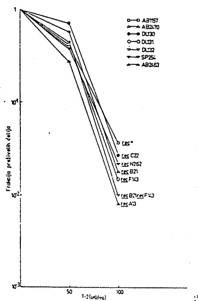
Sl. 2. Kriva preživljavanja rec sojeva tretiranih T-2 toksinom u trajanju od 40 min
