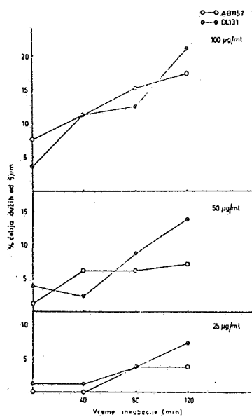
Sl. 4. Čelijska filamentacija indukovana T-2 toksinom
