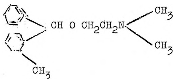
Strukturna formula orfenadrina
