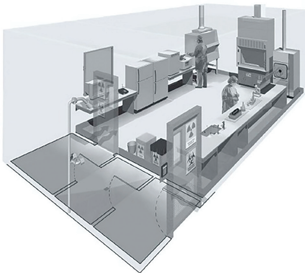
Slika 5. Prostorne karakteristike laboratorije nivoa 3 biološke bezbjednosti (Izvor: Niveles de Bioseguridad. Instituto técnico de bioseguridad y mantenimiento en el laboratorio, 24. 11. 2015. http://d11vm.blogspot.com/2015/11/niveles-de-bioseguridad-son-las.html (datum posljednjeg pristupa: 18. 1. 2024))
